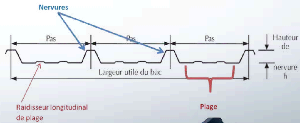
COUVERTURE ET BARDAGE BAC SEC
